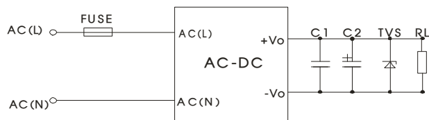
图 1：典型应用电路
