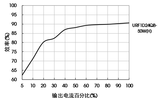
效率Vs输出负载 (标称输入)
